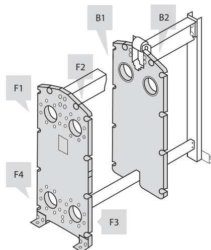
Верхнее расположение портов
