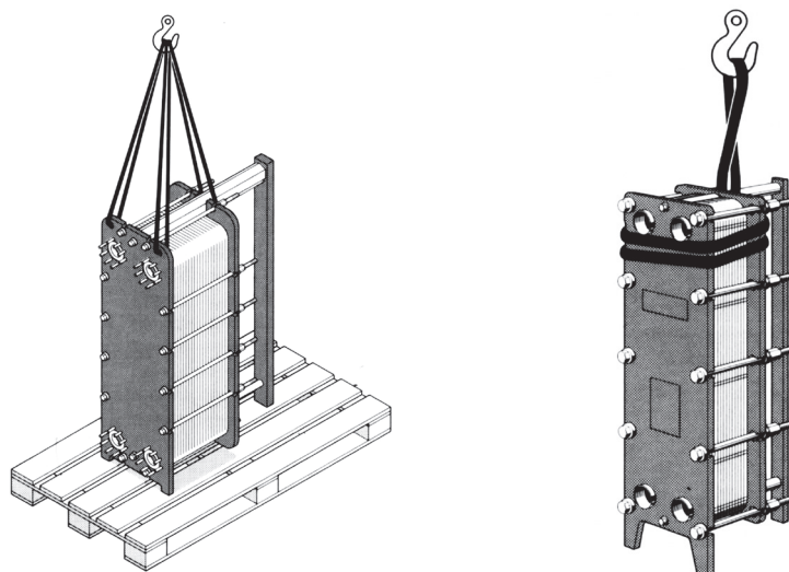
Строповка теплообменника с транспортировочными отверстиями
