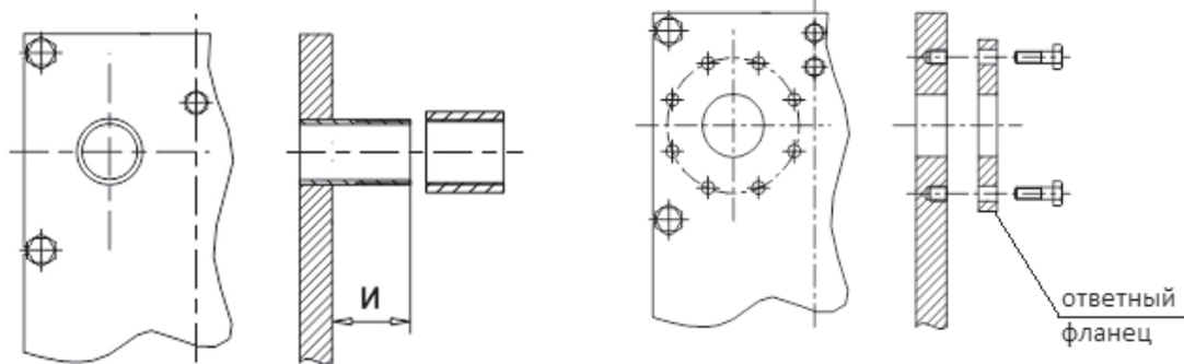
Резьбовой патрубков теплообменника
