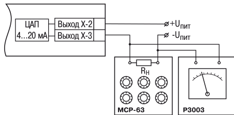
Рисунок 8.8 – Подключение ВУ1 типа У ( R_H=500\text{ Ом} )
