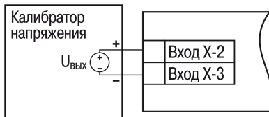
Рисунок 8.3 – Схема подключения при юстировке ТП
