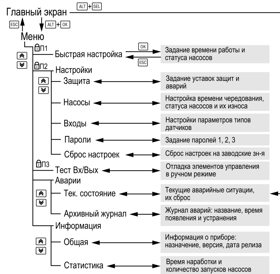
Рисунок 6.2 – Схема переходов по меню
