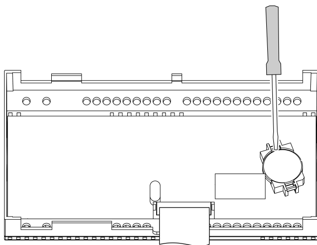
Рисунок 9.2 – Замена батарейки
