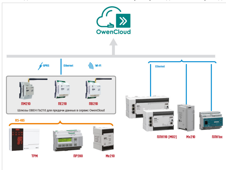
Рисунок 2.2 – Структурная схема подключения устройств пользователя к OwenCloud
