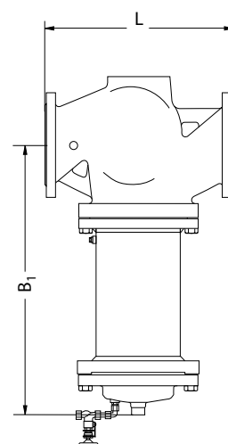
VFG2 Д y 50-250 с удлиненным штоком для T > 140 °C
